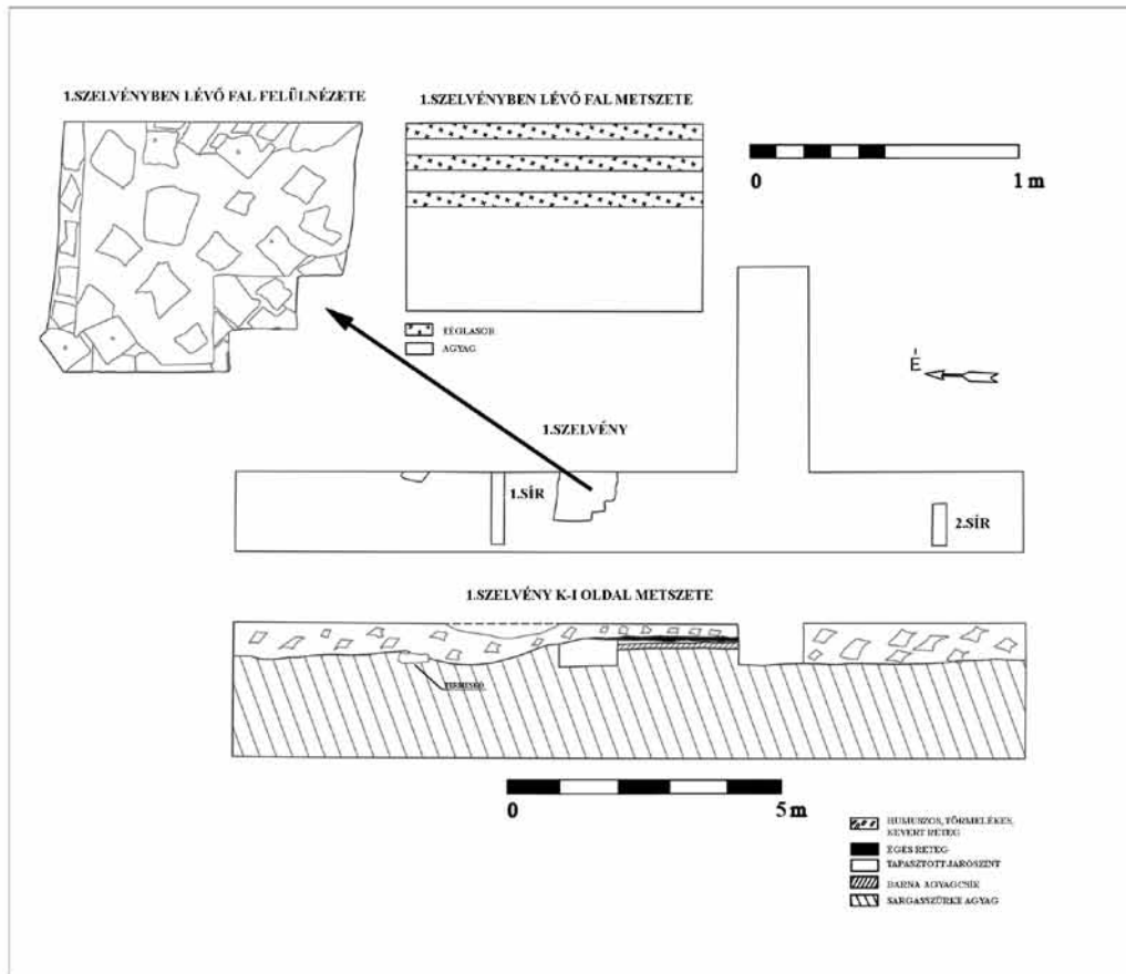
5. kép.: Újudvar - Gurda/Kolostordomb - az 1. szelvény alap- és metszetrajza a falszakasszal (GM Adattár: 357/26) Fig. 5.: Újudvar - Gurda/Kolostordomb - the ground plan and section of the profile Nr. 1. with the foundation of the wall (GM Adattár: 357/26)
