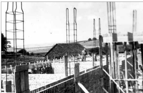
5. kép : Az erőmű épülete építés közben (1944)
