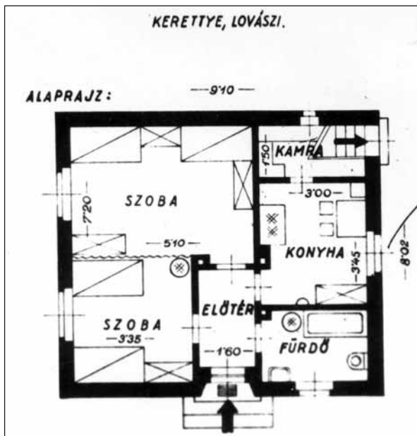
3. kép: Kétszobás munkáslakás alaprajza
