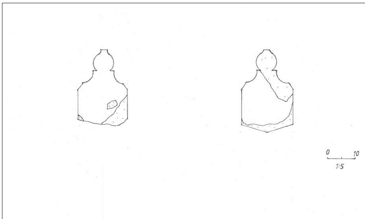
22. kép: Boltozati bordaprofil. (rajz: Klinger László, 2019.)
