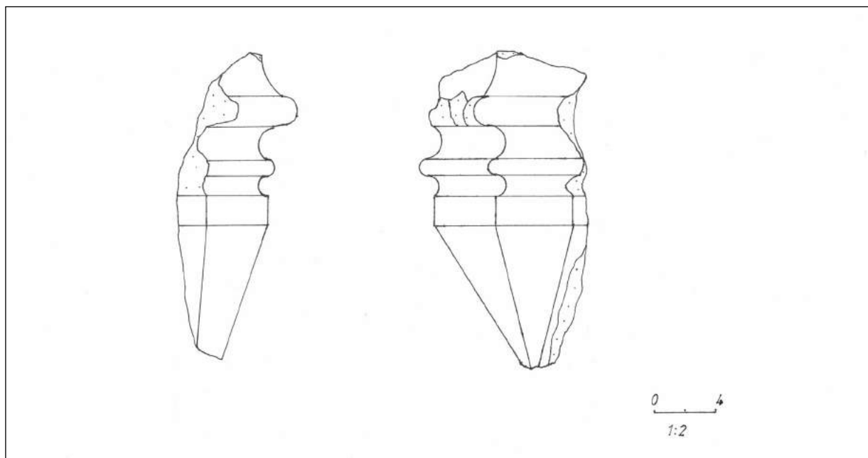
25. kép: Konzoltöredék. (rajz: Klinger László, 2019.)
