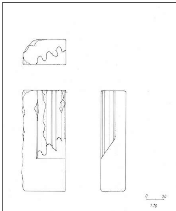
18. kép: Ajtókeret lábazati eleme. (rajz: Klinger László, 2019.)
