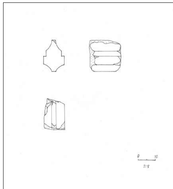
23. kép: Ablakosztó töredéke. (rajz: Klinger László, 2019.)
