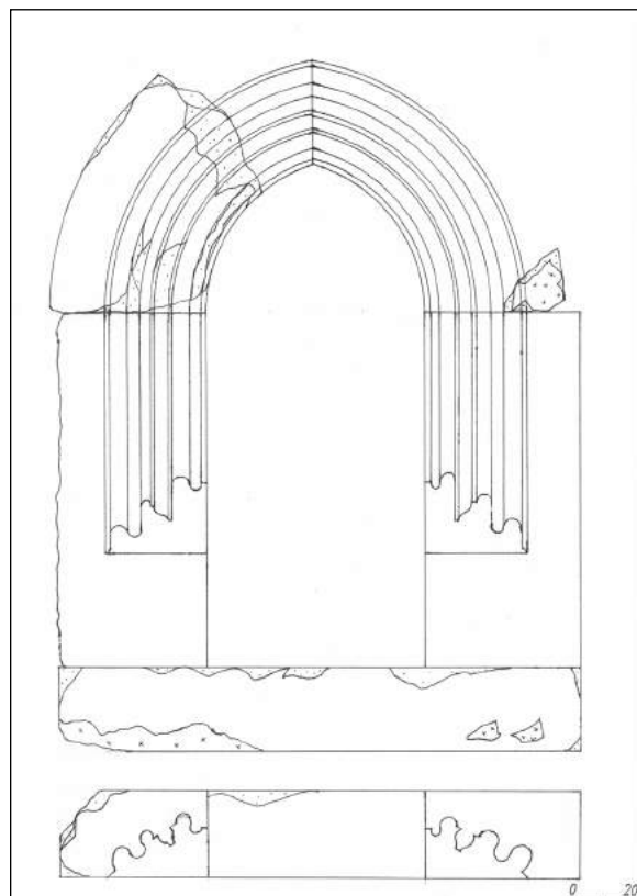
26. kép: A szentély északi falában nyíló ajtókeret rekonstrukciója. (rajz: Klinger László, 2019.)
