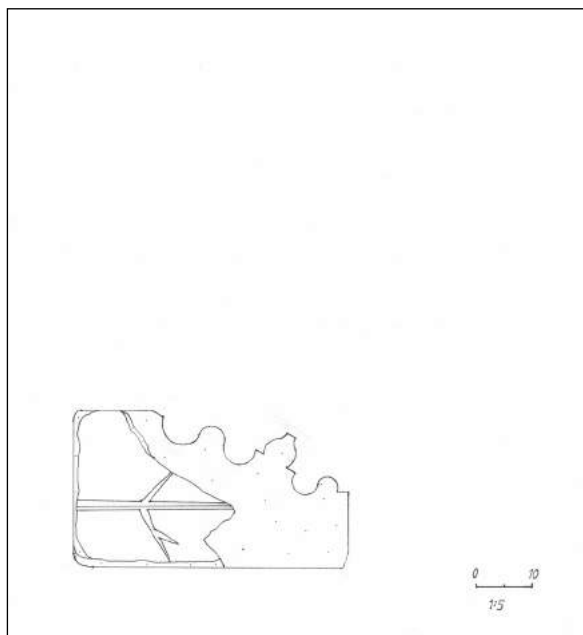
21. kép: Ajtókeret íves eleme. (rajz: Klinger László, 2019.)
