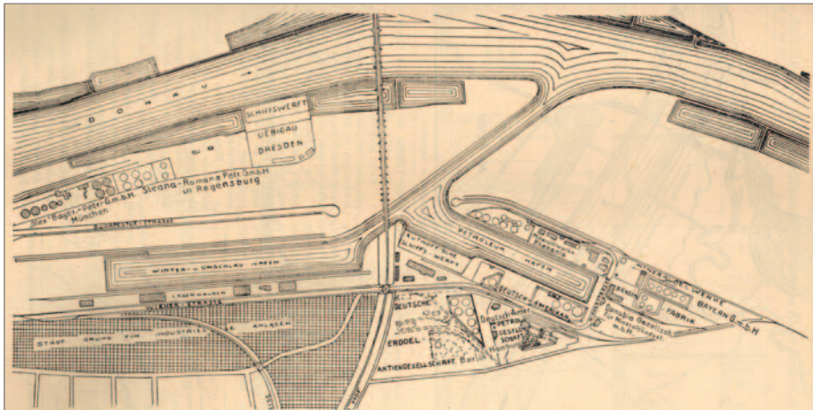
12. kép – A regensburgi petróleum- és téli-kikötő, valamint a kikötőnél megtelepedett olajipari cégek alaprajza
