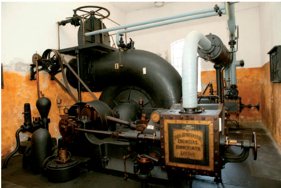
4. kép – Az első magyarországi szivattyútelep angol gépei a Heves megyei Sajfokon
